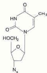
Zidovudine
